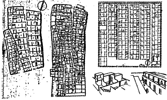
٣٣ منازل من الطوب اللين بالعمارة ودير المدينة - دولة حديثة
